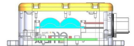
P2: screw+spacer+lens+spacer
